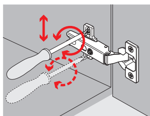
Nastavenie výšky
