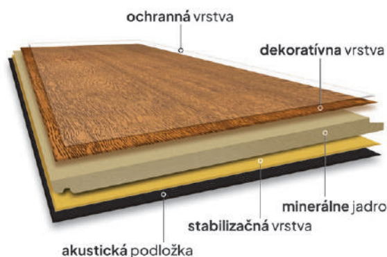
Štruktúra lamely (rez)
