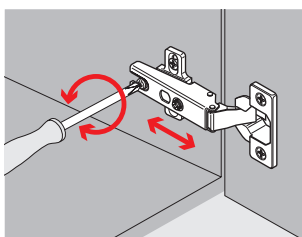
Nastavenie hĺbky
