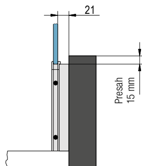
Detail A - pohľad spredu
