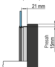
Detail A - pohľad spredu
