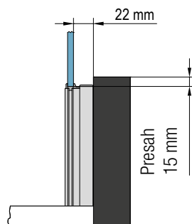
Detail A – pohľad spredu
