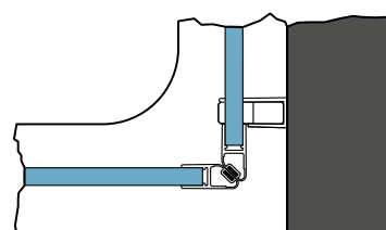
Detail A - pohľad shora
