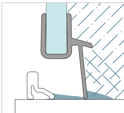
Čiastočne rámové zásteny s prahovou lištou
