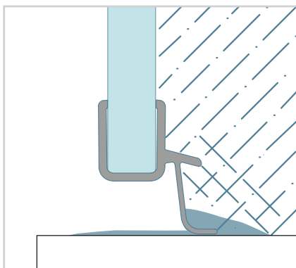
Bezrámové sprchové zásteny bez prahovej lišty
