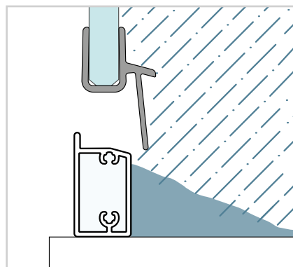
Rámové sprchové zásteny s rámovými profilmi
