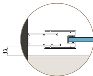
Obr. 1 Dvere, rohový vstup, štvrtkruh
